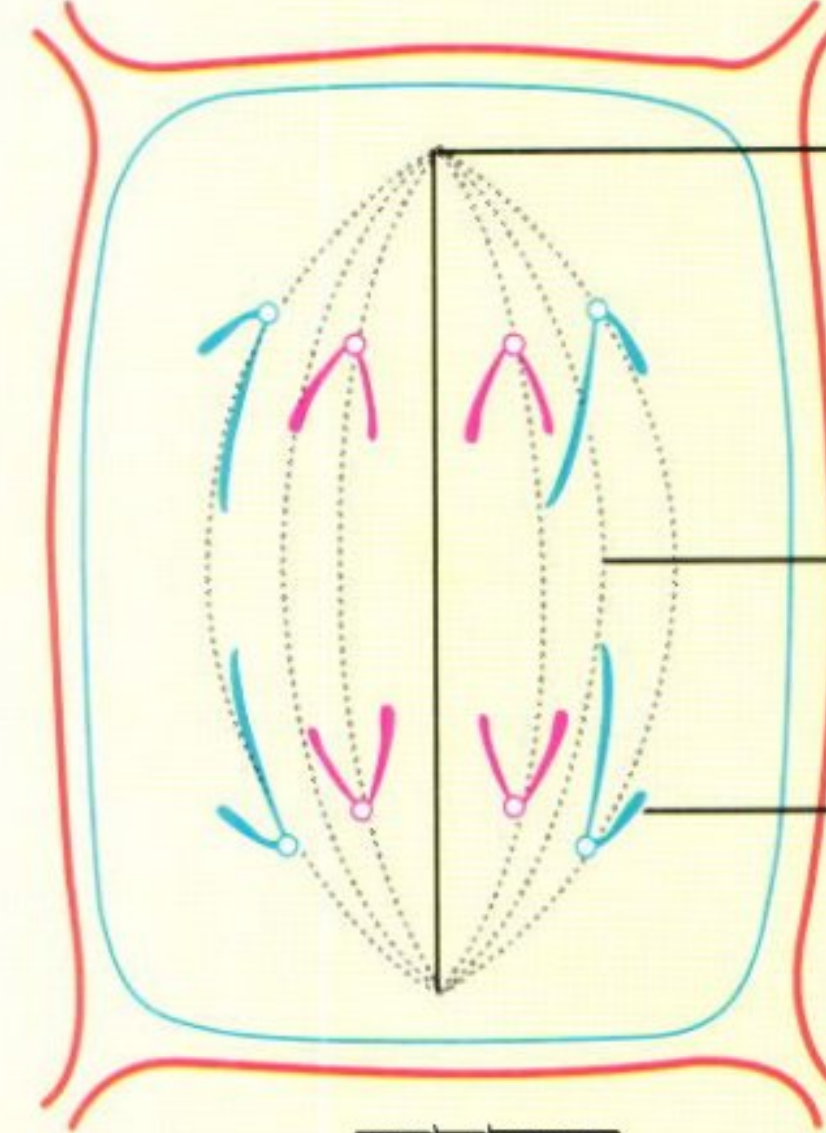
অ্যানাফেজ
