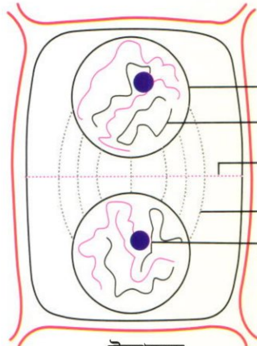
টেলোফেজ
