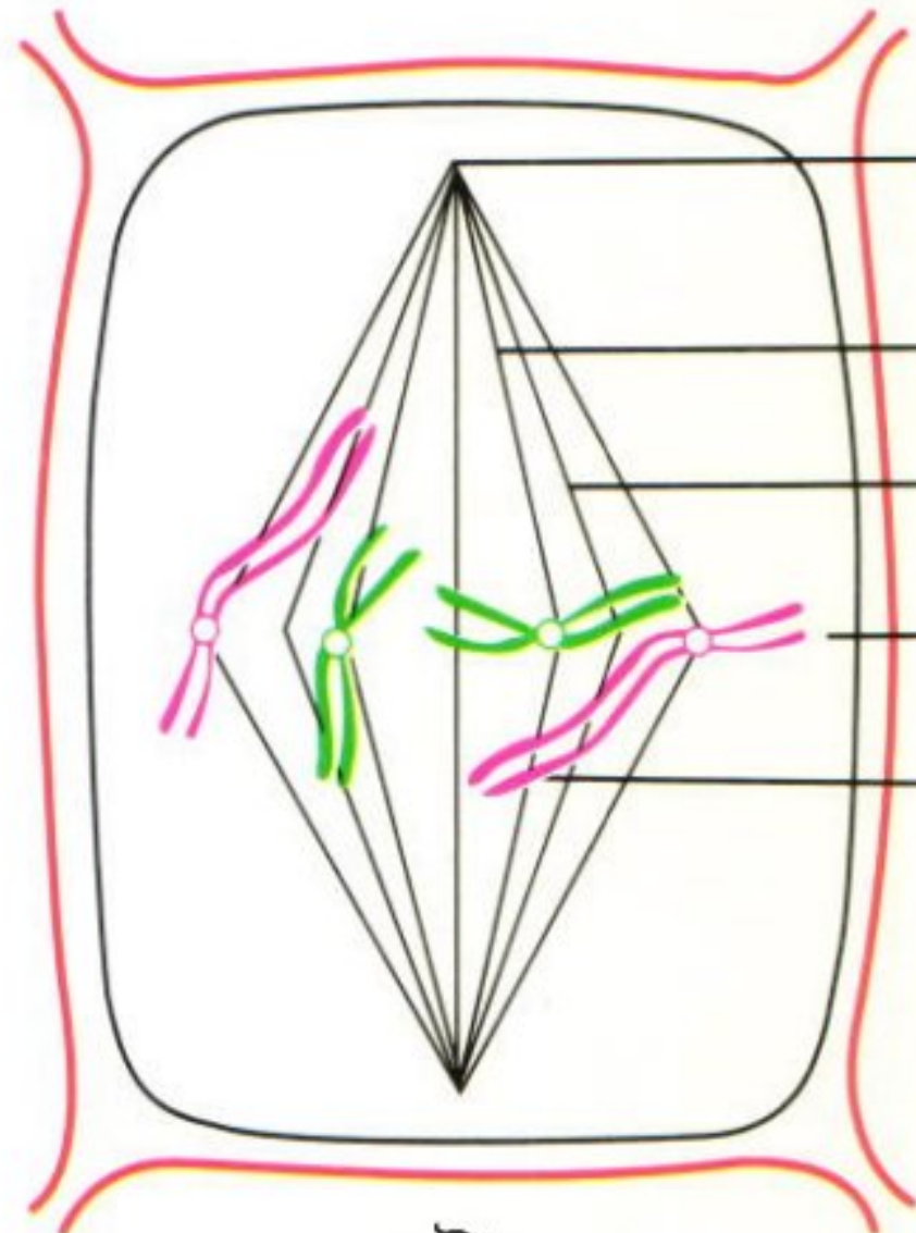
মেটাফেজ
