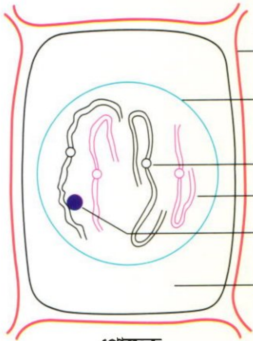
প্রোফেজ
