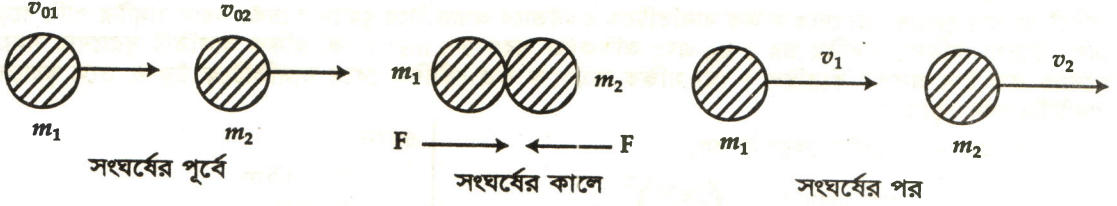
চিত্র ৪.৪৩ : পূর্ণ স্থিতিস্থাপক সংঘর্ষ।
