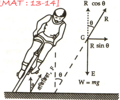
চিত্র ৪'৪১ : সাইকেল আরোহীর বাঁক নেওয়া।
